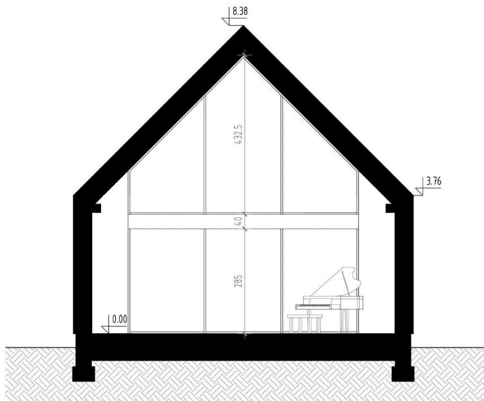
PRZEKRÓJ W STREFIE WYSOKIEGO SALONU
