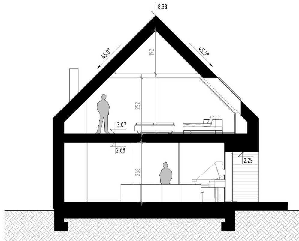
PRZEKRÓJ W STREFIE KUCHNI I SYPIALNI NA PODDASZU
